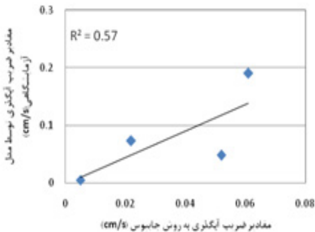
شکل ۳- همبستگی متوسط مقادیر مشاهداتی و روابط مختلف تعیین ضریب آنگوری خاک اشاع
