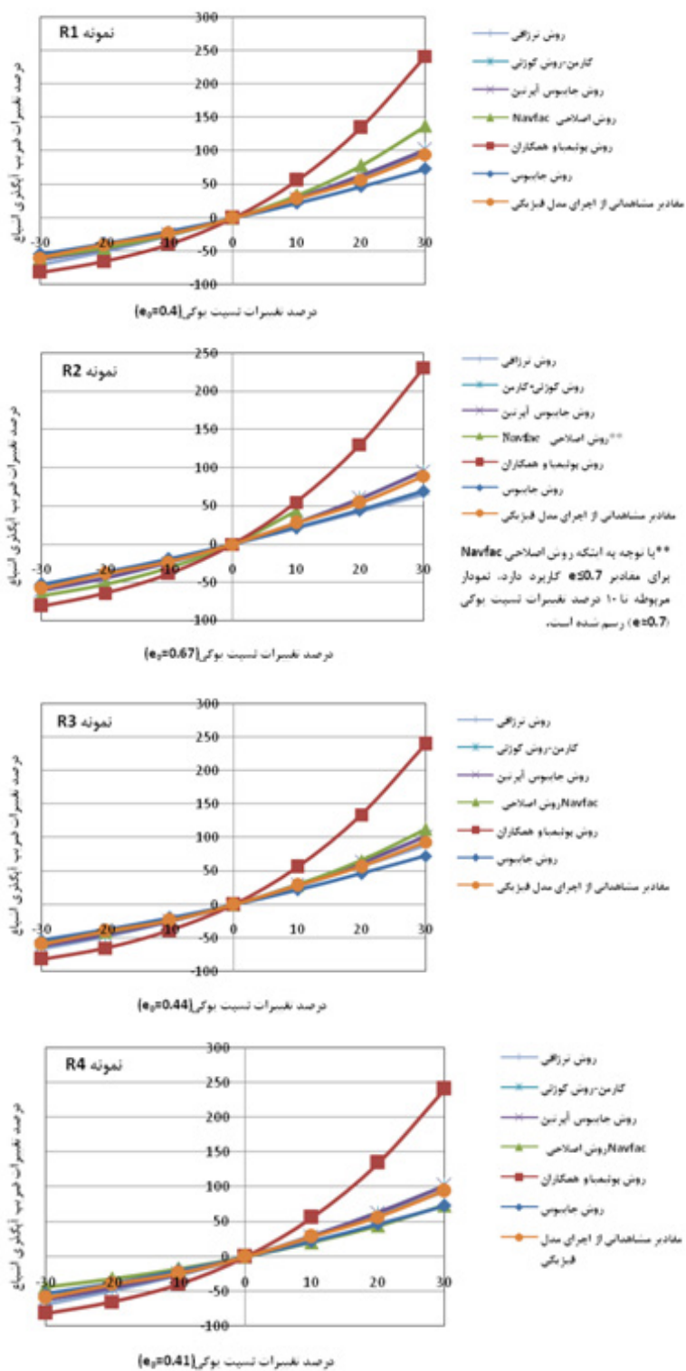
شکل ۸- درصد تغییرات ضریب آبگذری اشباع به صورت تابعی از درصد تغییرات نسبت بوکی برای نمونه‌های مختلف
