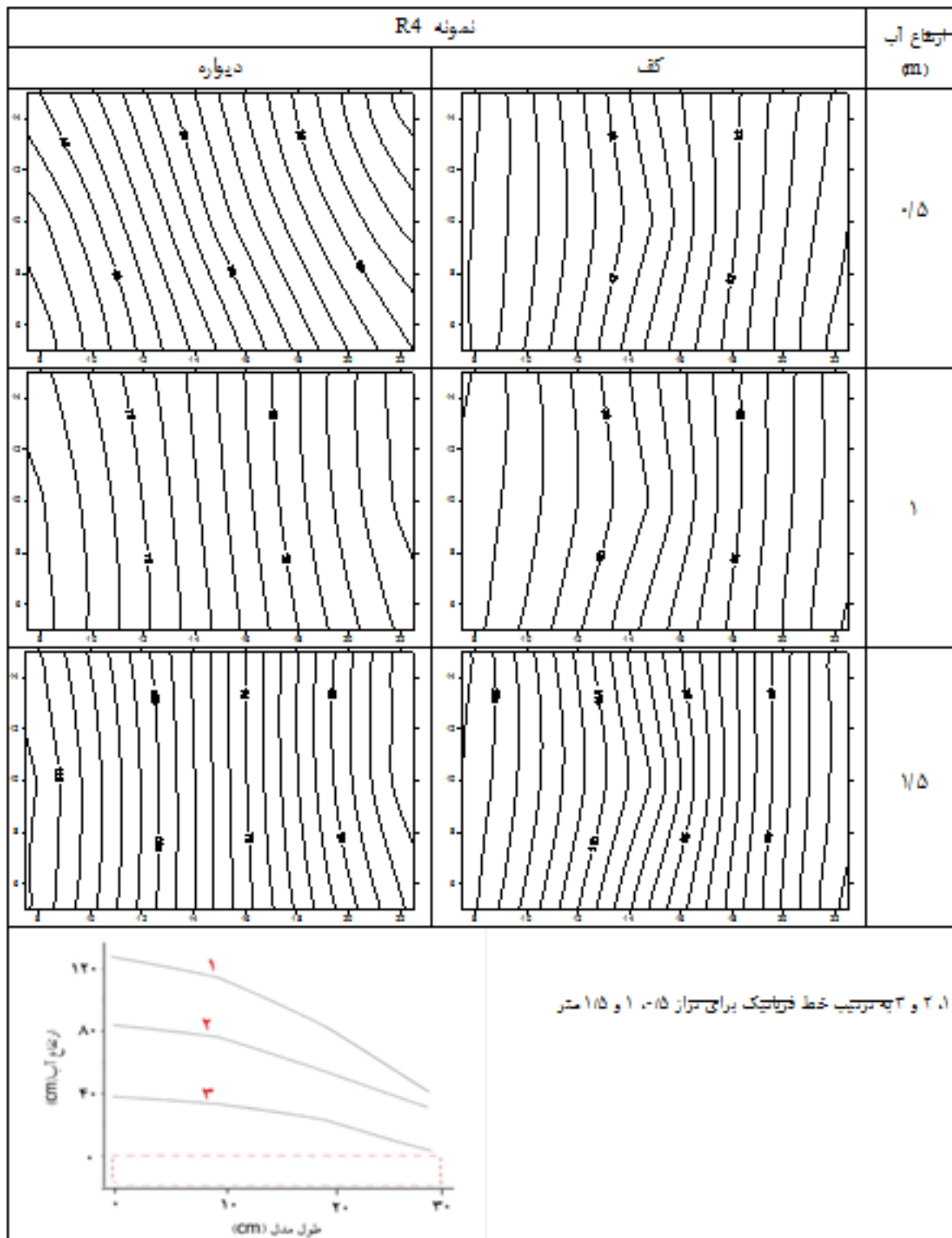
شکل ۷- وضعیت خطوط هم فشار و فریاتیگ برای نمونه R4 تحت ارتفاع‌های مختلف
