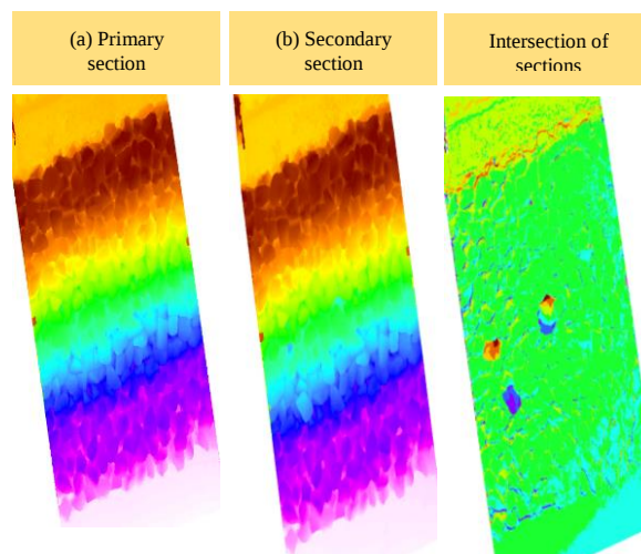
شکل ۴- ریخت‌شناسی مقطع P6 (a) قبل از تابش موج، (b) بعد از تابش موج، (c) تغییرات ریخت‌شناسی. Figure 4- Represents a) the profile shape before test, b) the profile after test, c) the intersection of profiles after the 9 th test.
