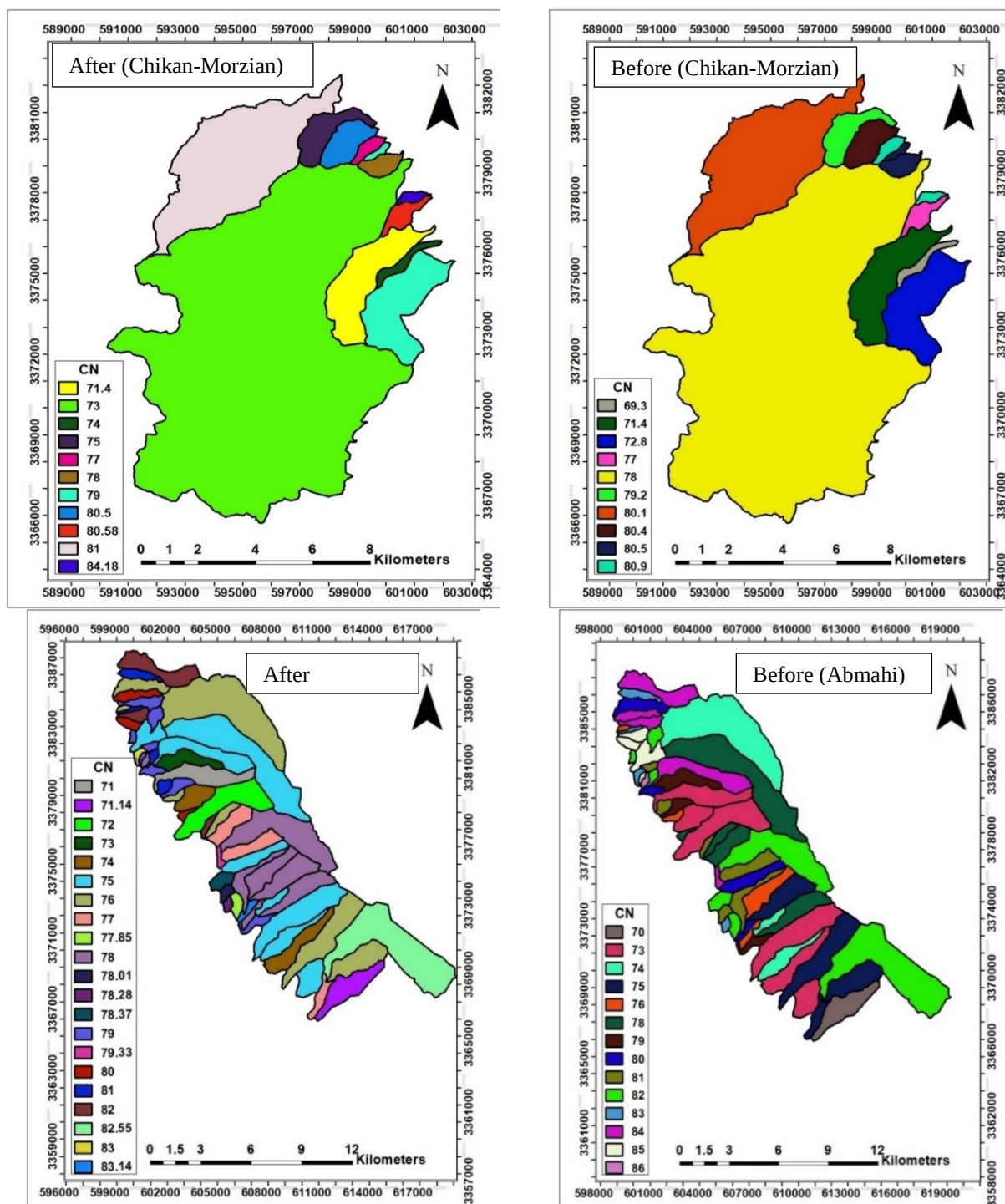
شکل ۲- نقشه CN زیرآب‌خیزهای چیکان - مورزبان و آب‌ماهی در شرایط قبل و بعد از اقدامات آبخیزداری. Figure 2- CN map of the Chikan-Morzian and Ab-Mahi sub- watershed before and after the watershed management measures.
